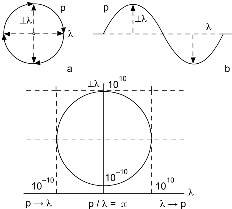
Abb. 5 Eine vergleichende Gegenüberstellung der Wellenformen. Sowohl sphärische Welle (a) als auch ausgedehnte Welle (b) können mit gleichen Zustandsgrößen beschrieben werden ( p , \lambda , \perp\lambda ). Ein Diagramm unten veranschaulicht die Verhältnisse zwischen diesen Zustandsgrößen.
