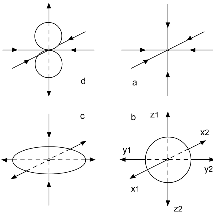
Abb. 4 Koordinatensysteme in einem multifocalen Universum. Jeder Punkt des Raumes stellt eine singulare Potenz dar (a entspricht etwa den Knotenpunkten einer stehenden Welle), die verschiedene Konformationen annehmen kann: Aus dem Null-Punkt kann infolge der Ausdehnung eine Form entstehen (c und b entsprechen den 2-D- und 3-D-Flächen); die Ausdehnung weicht der Unterteilung (d). Die Superposition des Raumes entsteht infolge überlappender und aufsteigender Kreise der Wechselwirkungen, wo es keine Unterbrechung zwischen Mikro- und Makrozuständen gibt. Die Zustandsdauer wird als Zeiteinheit definiert, die Zeit erscheint als eine permanente Größe, die aus einzelnen Zuständen
