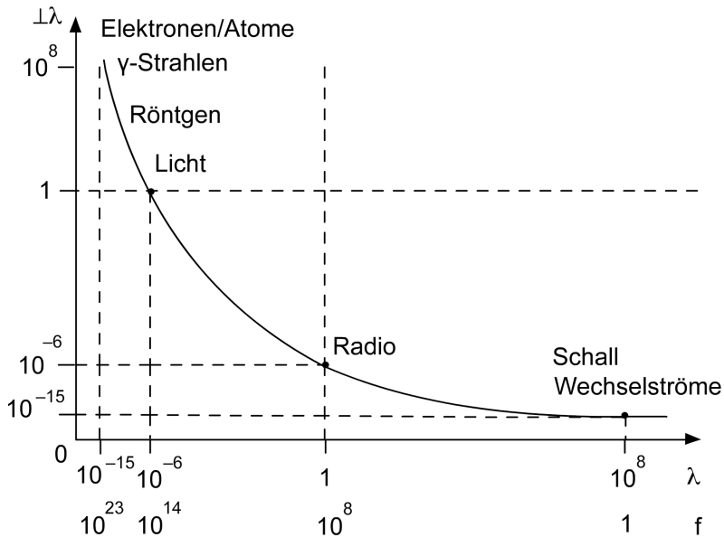
Abb. 8 Das geometrische Wellen-Spektrum. Die Verhältnisse zwischen den Wellenklassen sind in einem Diagramm zusammengefasst, und beziehen sich auf die Positionen, wo die Maßgrößen \lambda und \perp\lambda jeweils den Wert von 1 annehmen. Das Spektrum bekommt damit die Symmetrie-Achsen, die den Raum dieses Diagramms unterteilen, was bei einer traditionellen Darstellung nicht zum Vorschein kommt.
