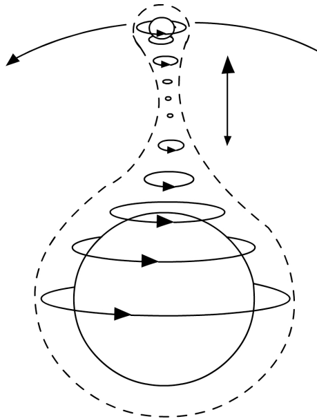
Abb. 10 Diagramm zeigt 2 Himmelskörper als ein reziprokes isoliertes System. Die Hilfslinien verdeutlichen topologische Konfiguration 2/3 D, die Verteilung von Wechselwirkungen, und die Änderungen der Raumstruktur, die man als Bewegungen wahrnimmt.
