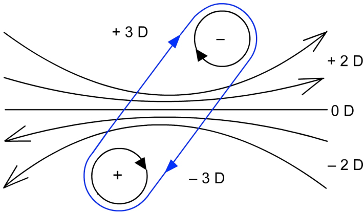
Abb. 1 Die Verhältnisse zwischen Dimensionen in Bezug auf das Paradigma aufgeteilter Räume. Die Phasen eines Raumes trennen sich infolge der Raumpolarisation; an der Grenze entsteht eine selbständige Struktur, die Membrane.
