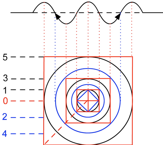
Abb. 6 Der Proportionsvergleich zwischen einem Kreis bzw. einer Sphäre und einer harmonischen Schwingung. Die Verdoppelung der Kreisflächen stimmt mit der Periodizität einer Welle überein. Die Elementarquadrate und der Elementarkreis sowie die Kreis- und Hilfslinien, die dieser Verdoppelung entsprechen, sind farblich markiert (schwarz steht für ungerade, blau für gerade Werte der Ordnungszahl n ).
