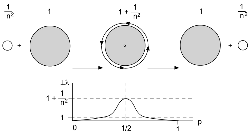
Abb. 7 Eine verallgemeinerte Darstellung der Periodizität. Während das Atom eine elementare Quantität aufnimmt (Absorption), dehnt es aus (Ausdehnung wenn n > 1 , Unterteilung wenn n = 1 ). Bei 1/\lambda = 1 befindet
